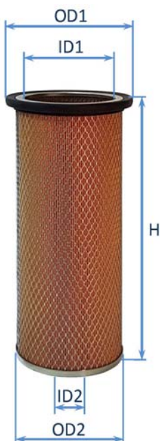
GD2404 Secondary air filter (هوای درونی)
