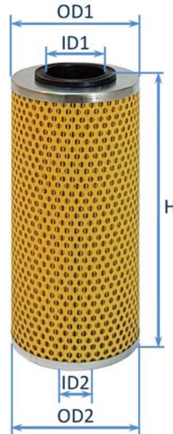
GE2254 Hydraulic oil filter (روغن هیدرولیک)
