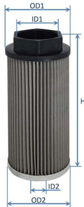
GE2255 Hydraulic oil filter (روغن هیدرولیک)
